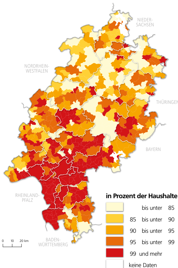
Abbildung 51 Mobilfunkverfügbarkeit LTE \geq 6 Mbit/s 2019 in Prozent der Haushalte
